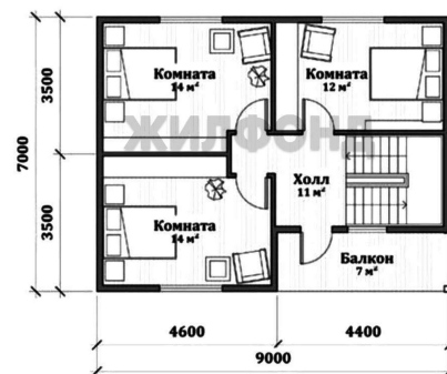
План 2-ого этажа
