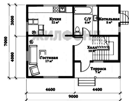
План 1-ого этажа
