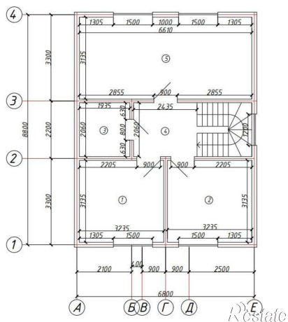
План 2-ого этажа
