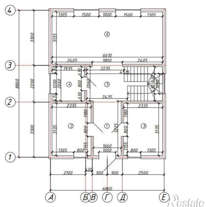
План 1-ого этажа
