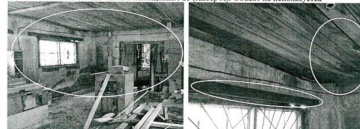
Следы загнивания стены из арболитовых блоков; отклонение от вертикали наружных деревянных ограждающих конструкций в помещении № 6/а (Литер а)
